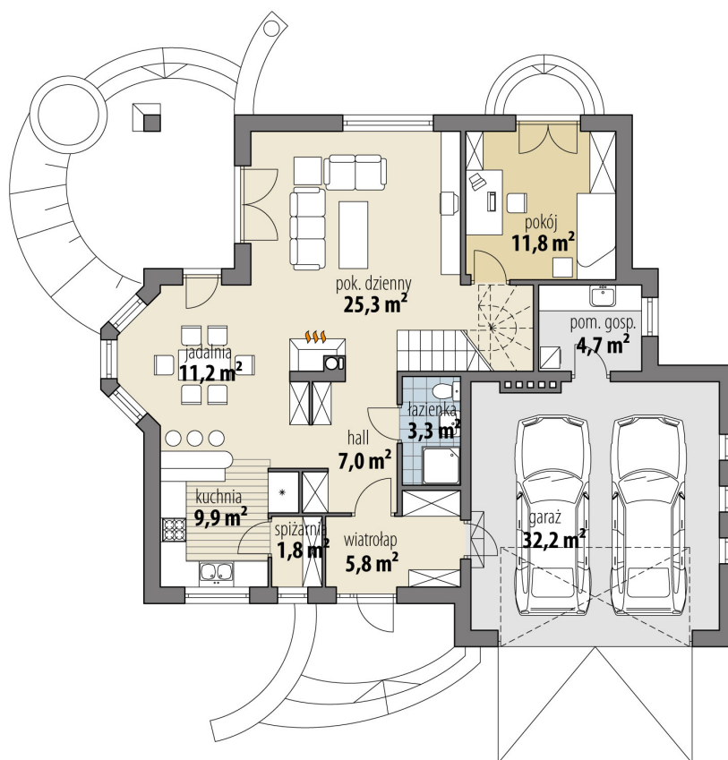
RZUT PARTER
