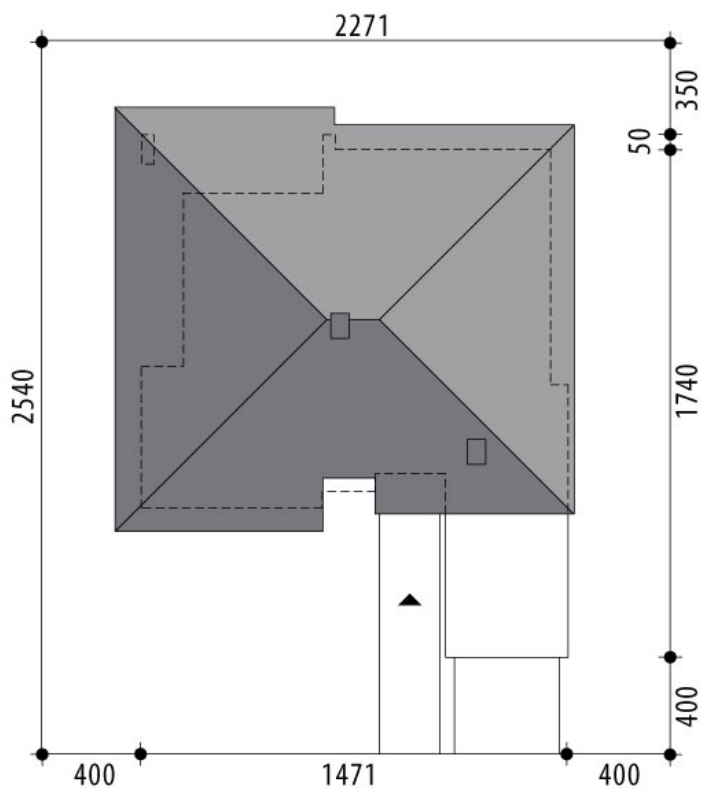
RZUT DZIAŁKI
