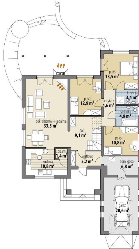
RZUT PARTER
