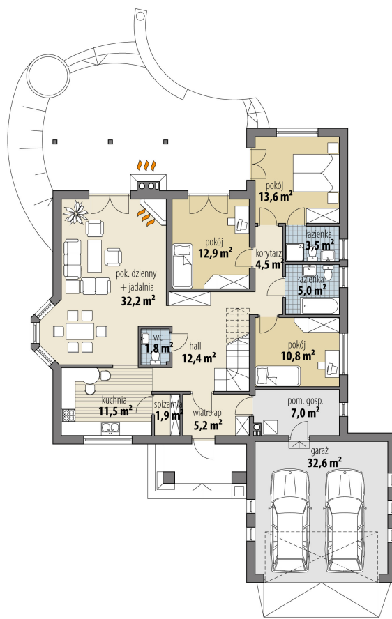
RZUT PARTER
