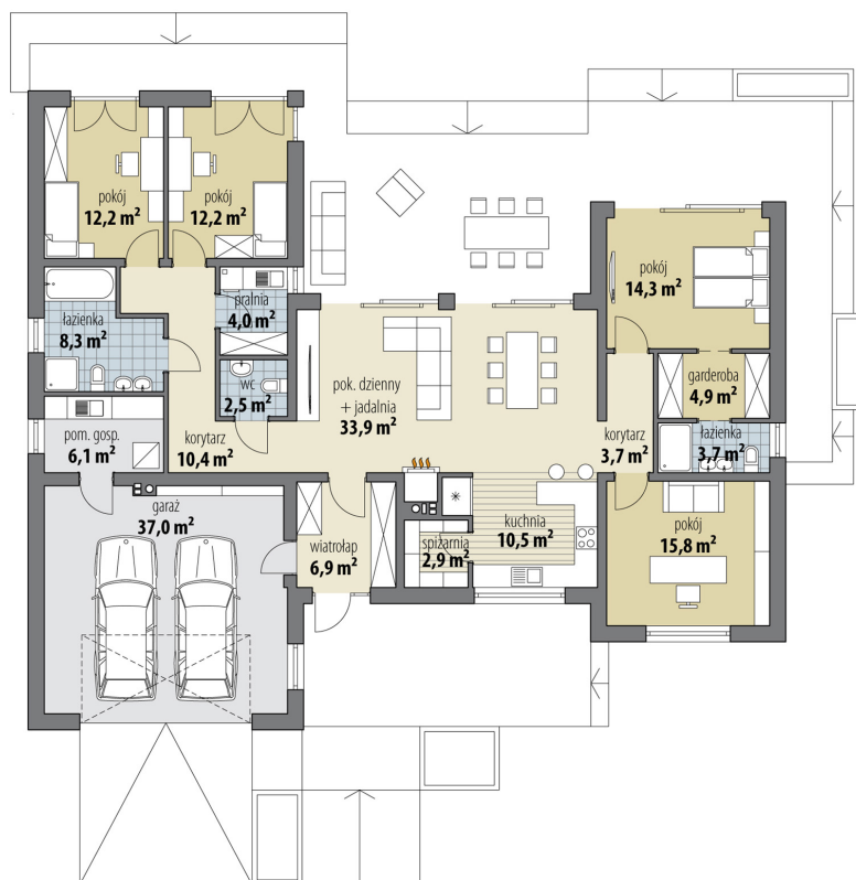
RZUT PARTER
