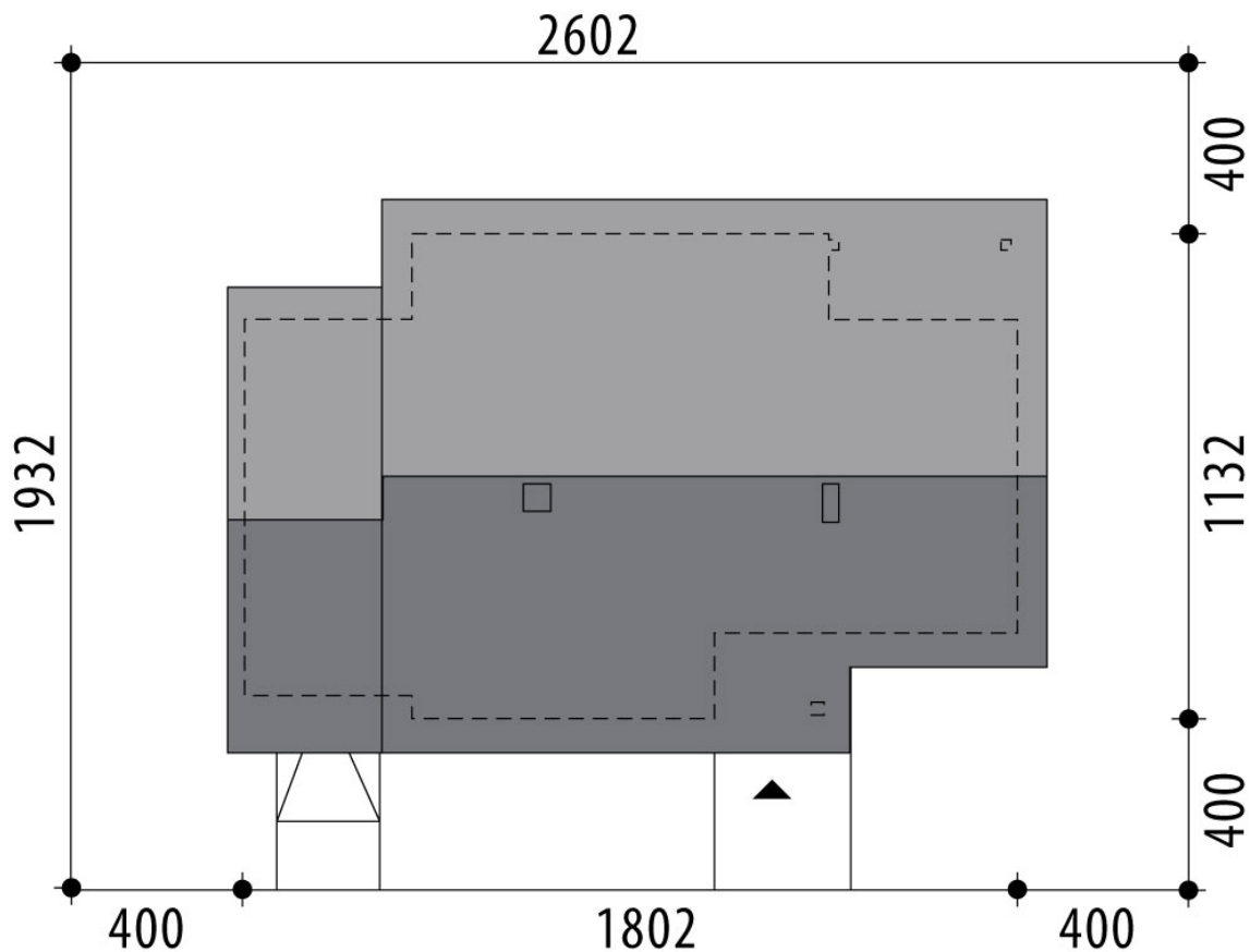
RZUT DZIAŁKI
