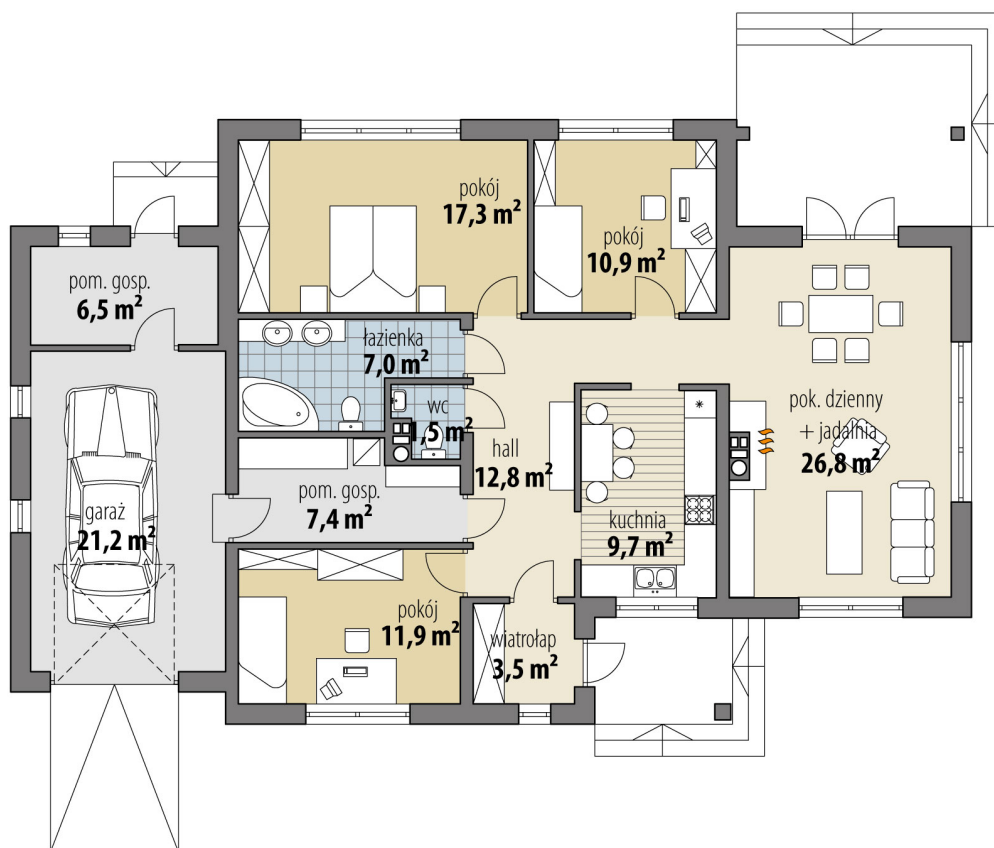
RZUT PARTER
