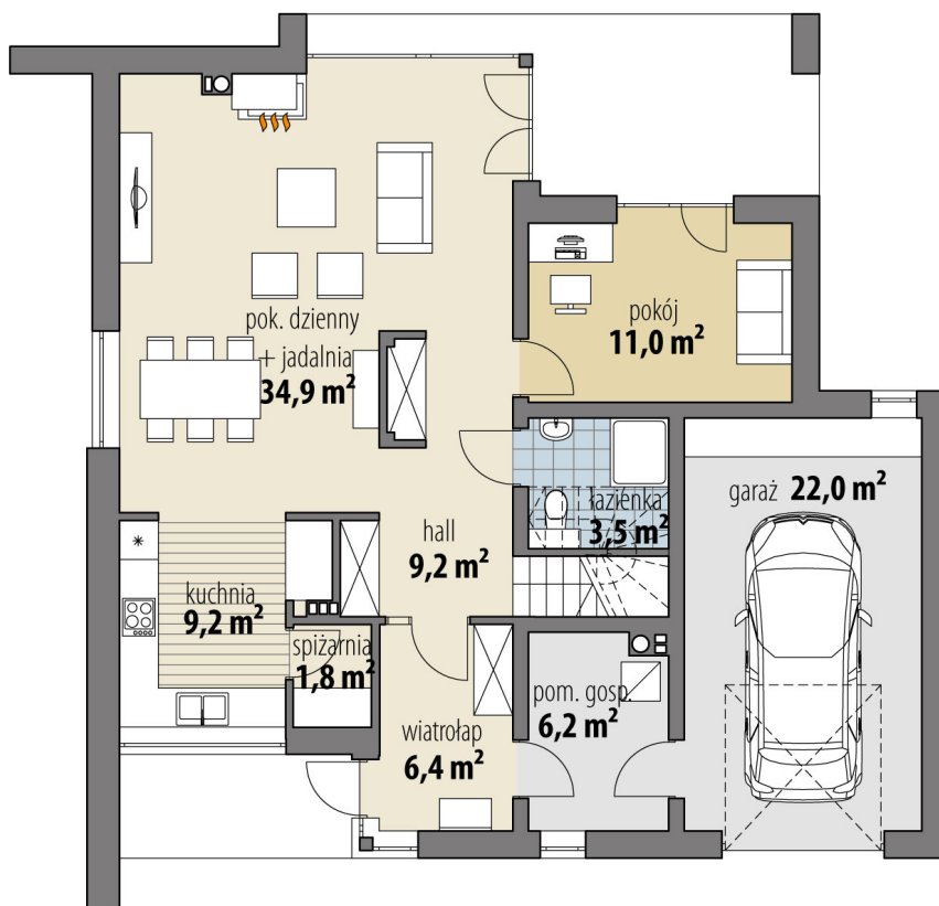
RZUT PARTER
