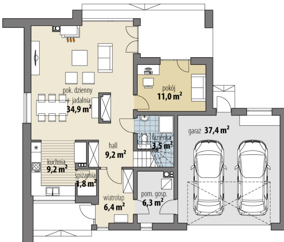
RZUT PARTER
