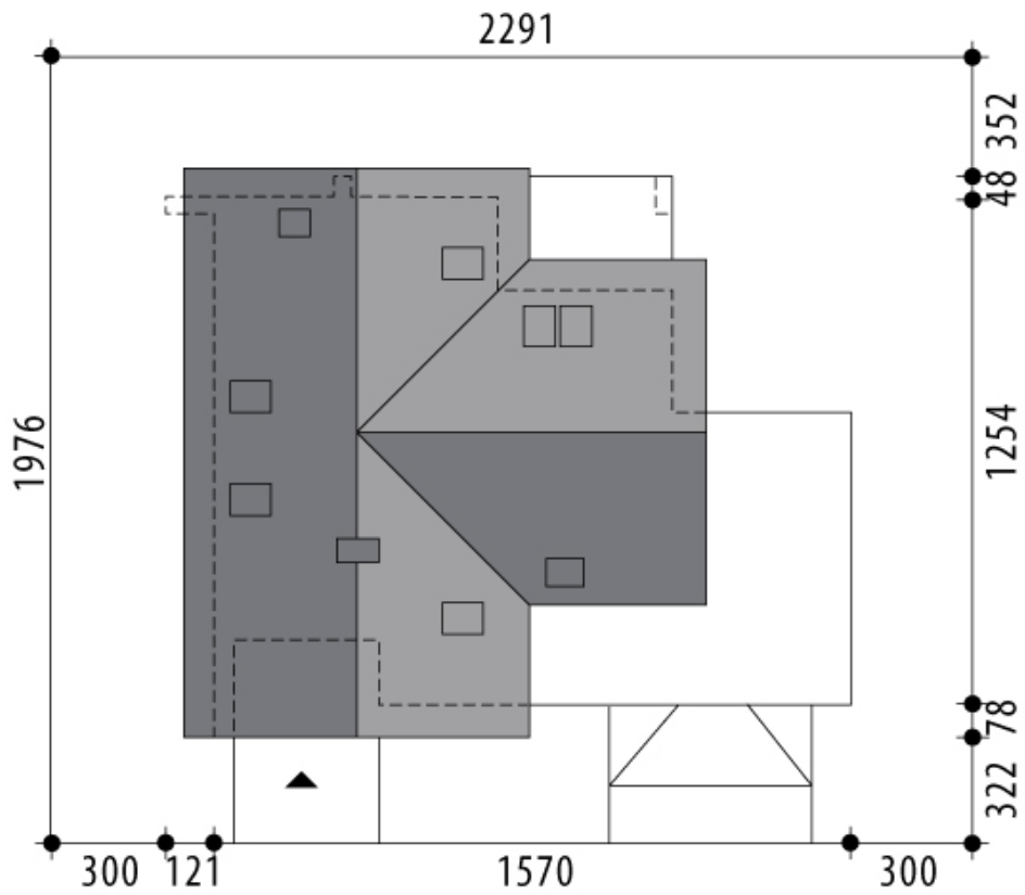
RZUT DZIAŁKI
