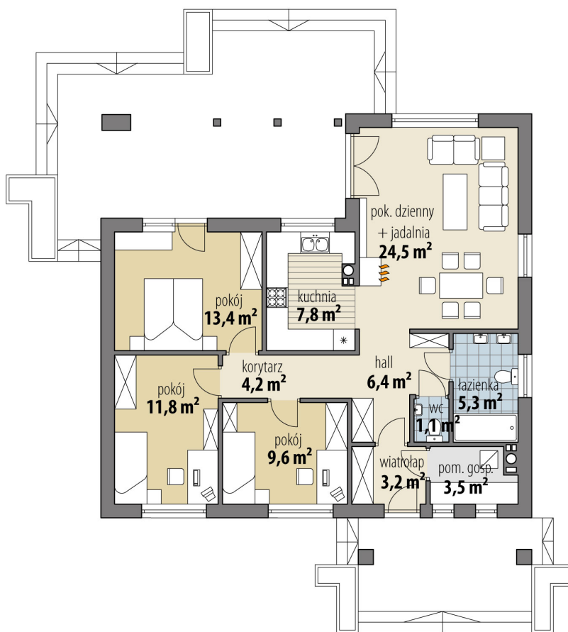
RZUT PARTER
