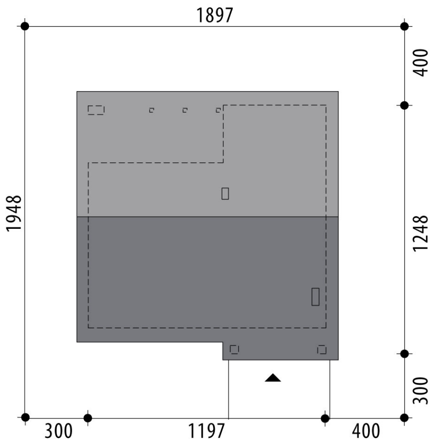
RZUT DZIAŁKI
