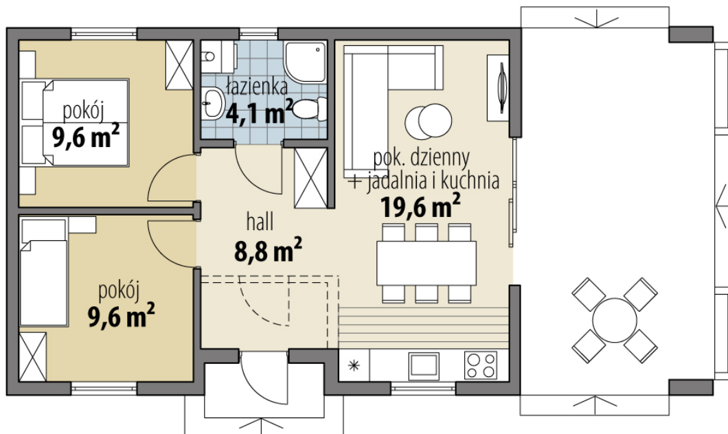
RZUT PARTER
