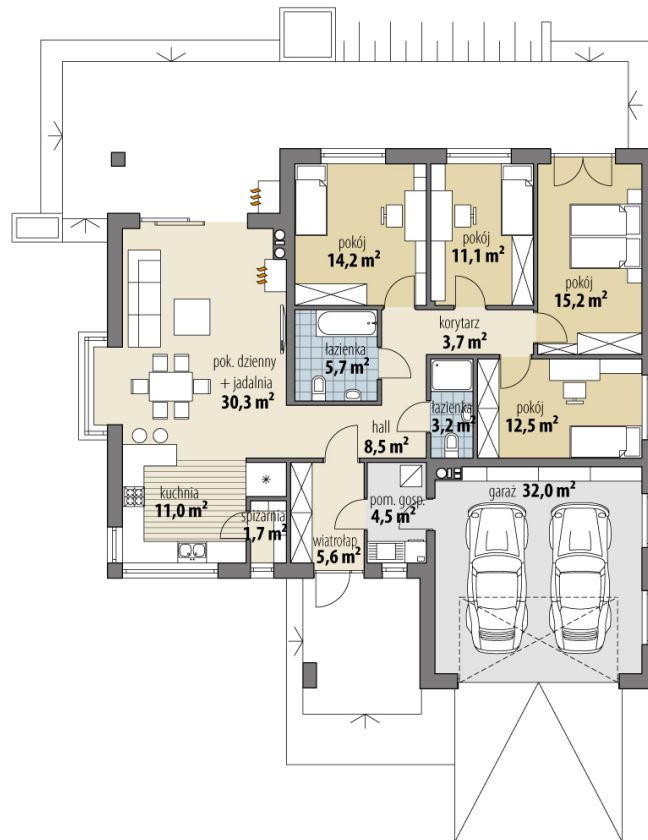
RZUT PARTER
