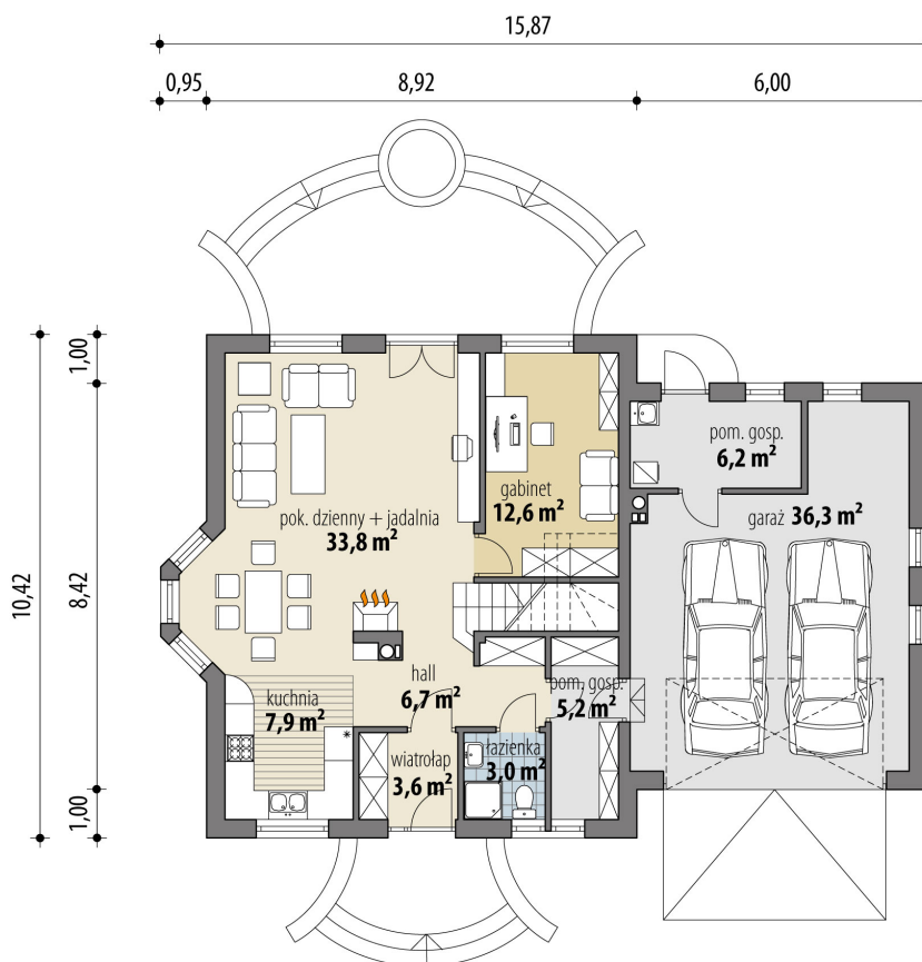
RZUT PARTER
