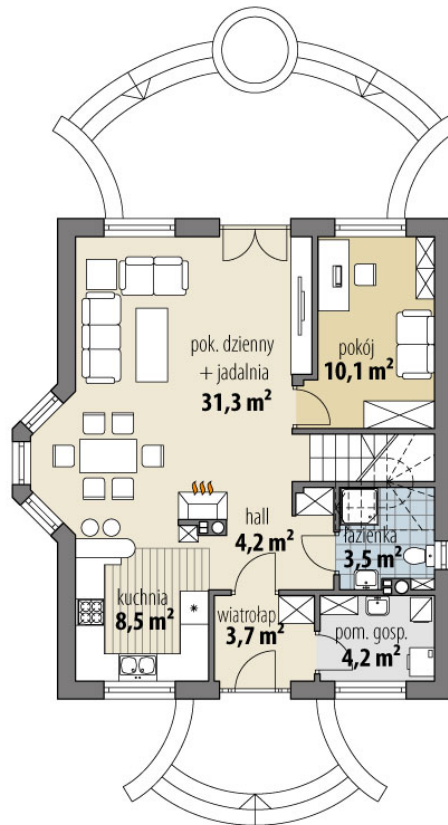
RZUT PARTER
