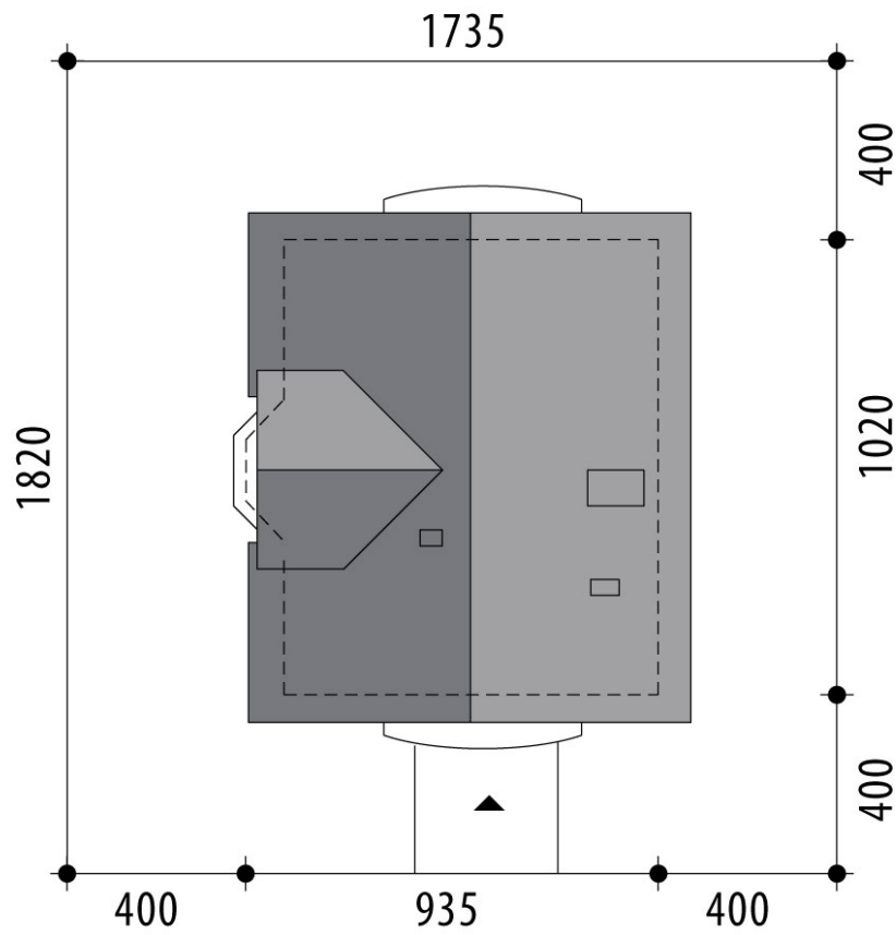
RZUT DZIAŁKI
