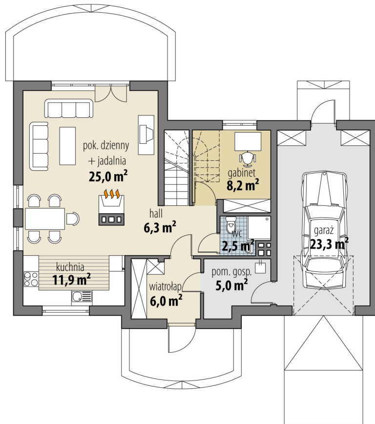
RZUT PARTER
