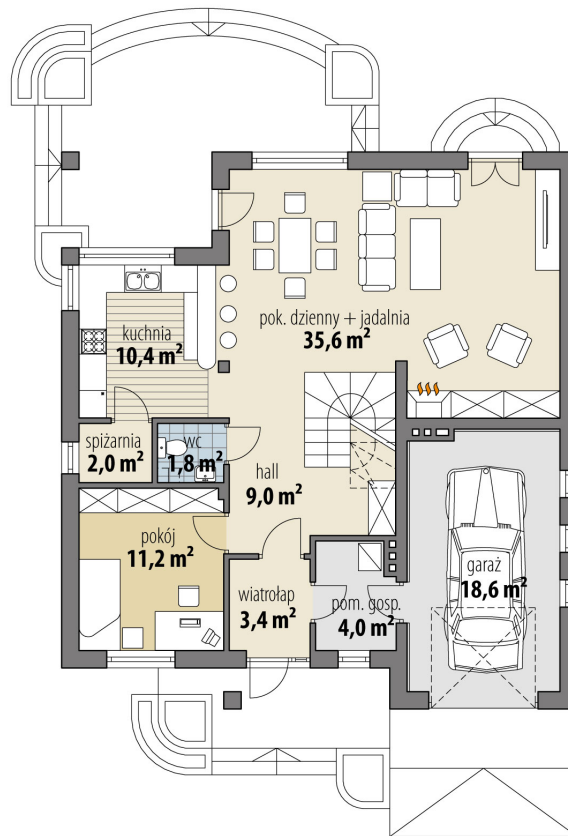
RZUT PARTER
