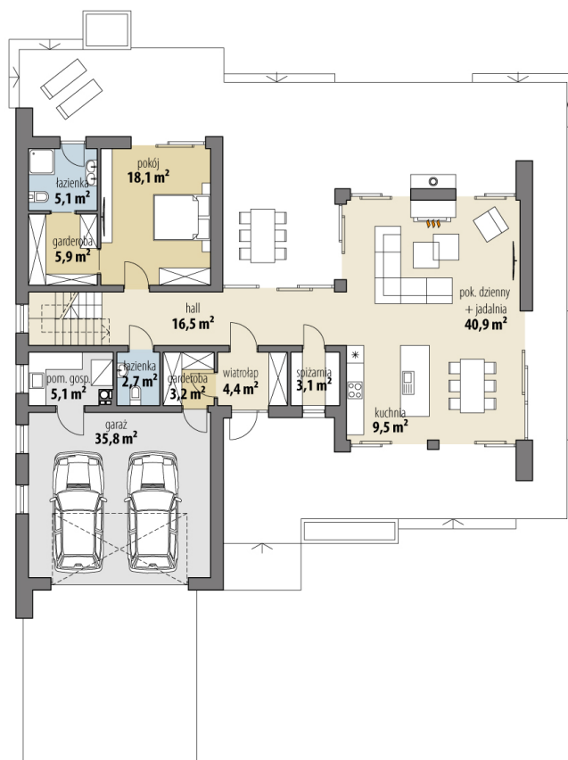
RZUT PARTER
