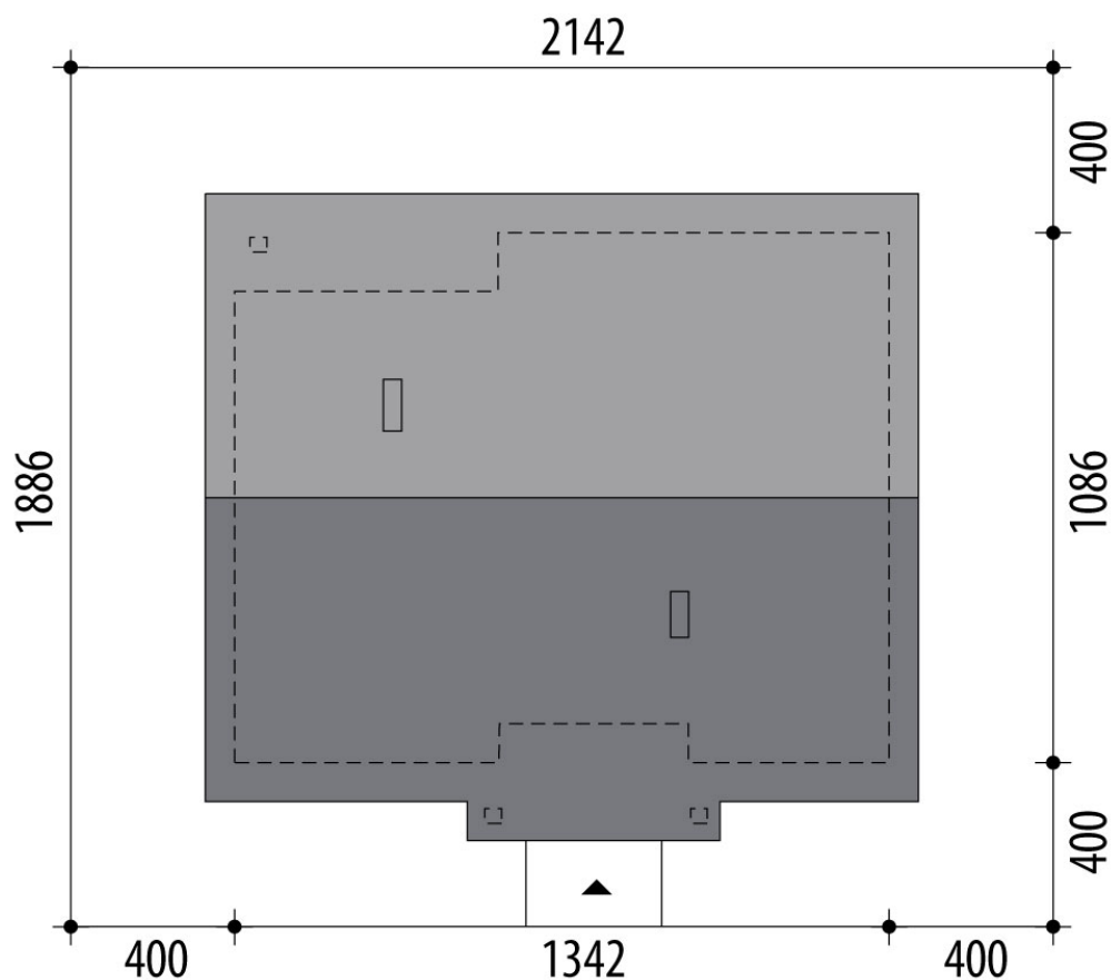
RZUT DZIAŁKI
