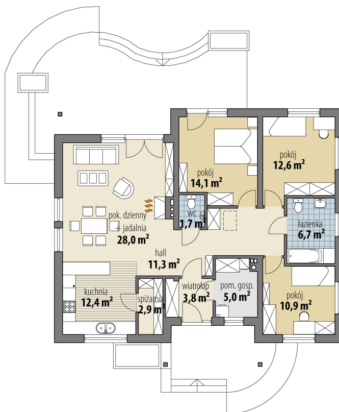
RZUT PARTER
