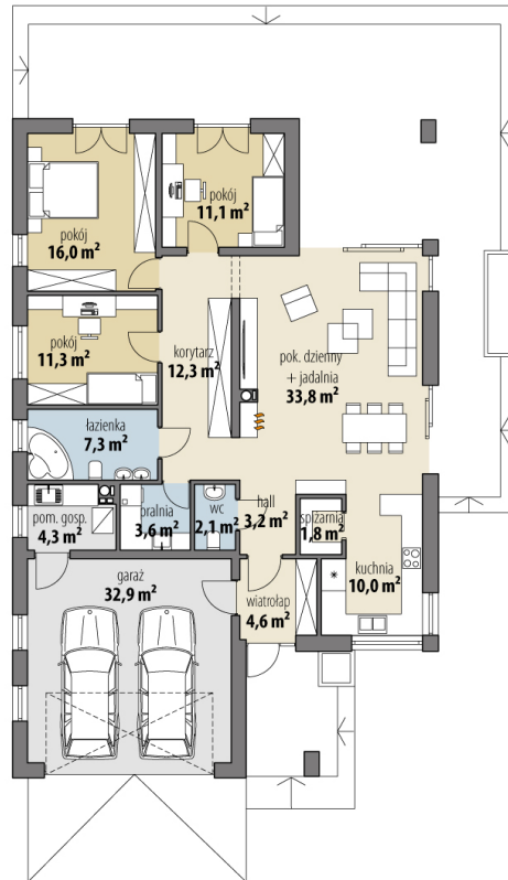
RZUT PARTER
