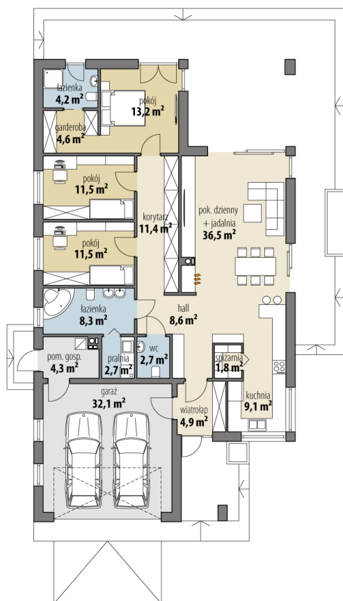
RZUT PARTER
