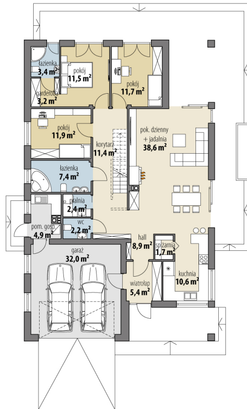
RZUT PARTER
