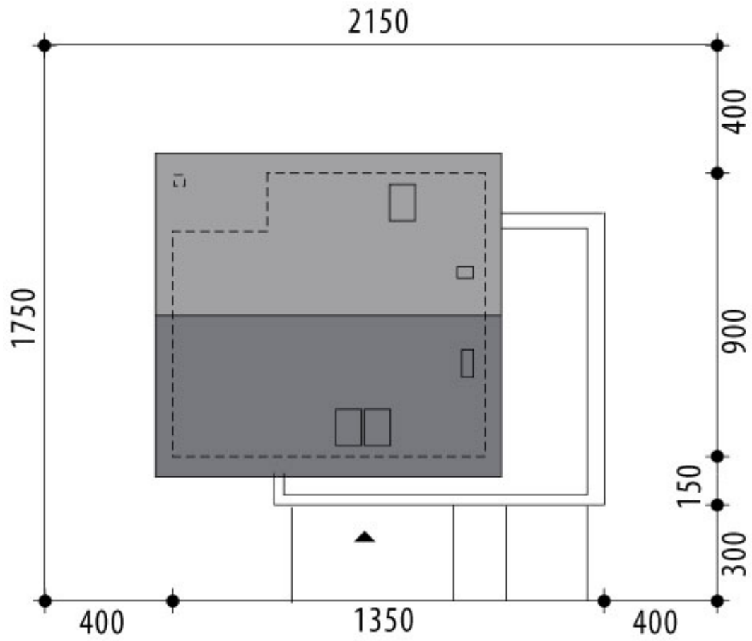
RZUT DZIAŁKI
