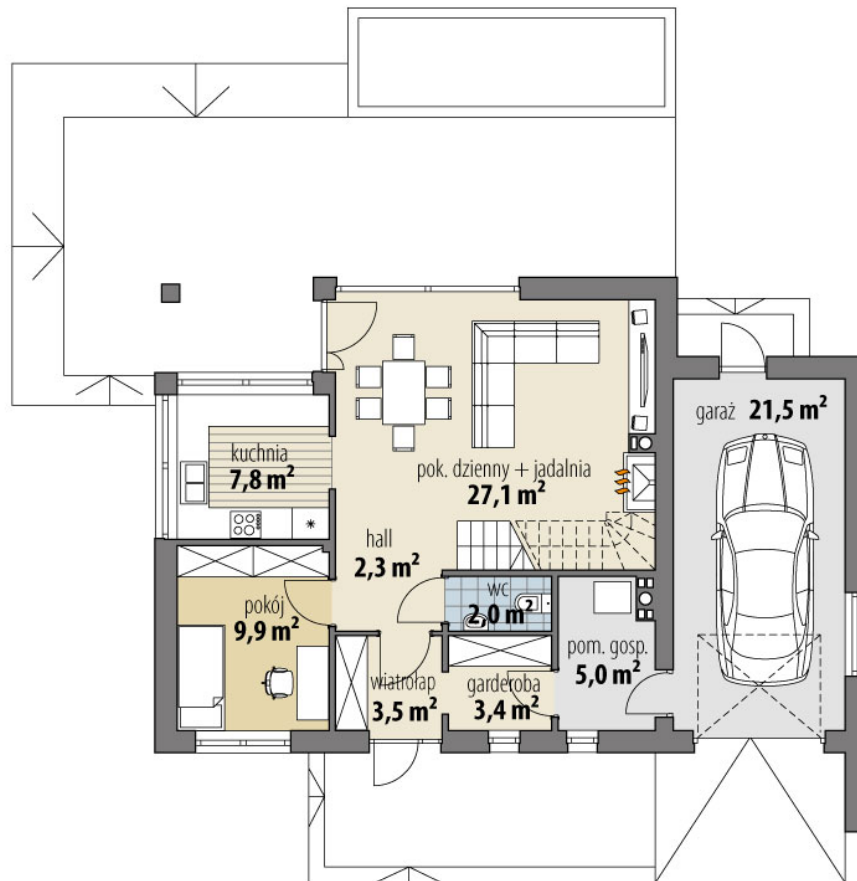
RZUT PARTER
