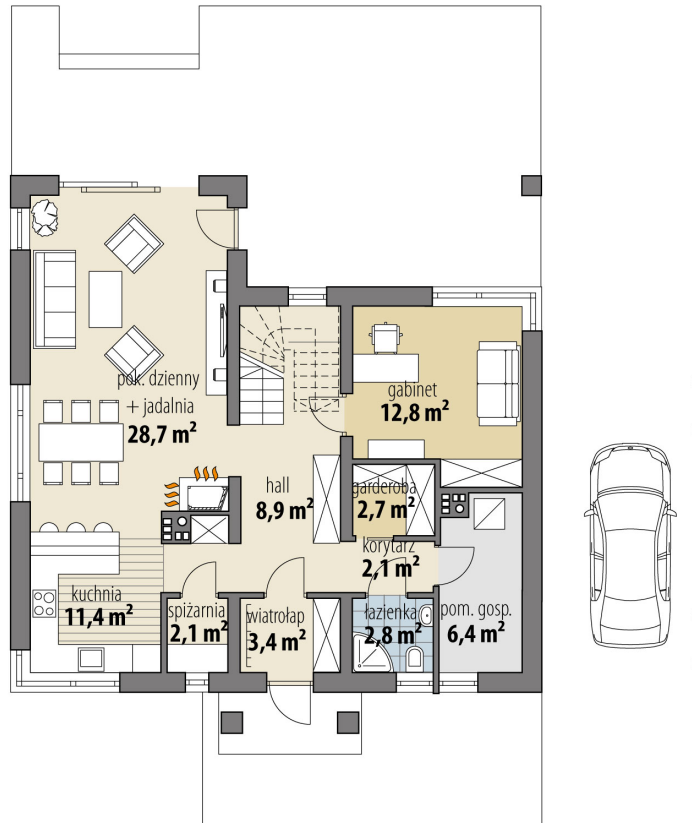
RZUT PARTER
