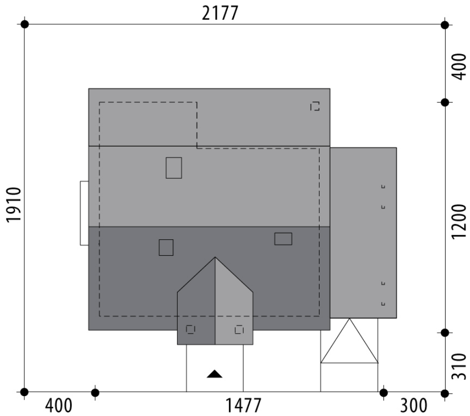
RZUT DZIAŁKI
