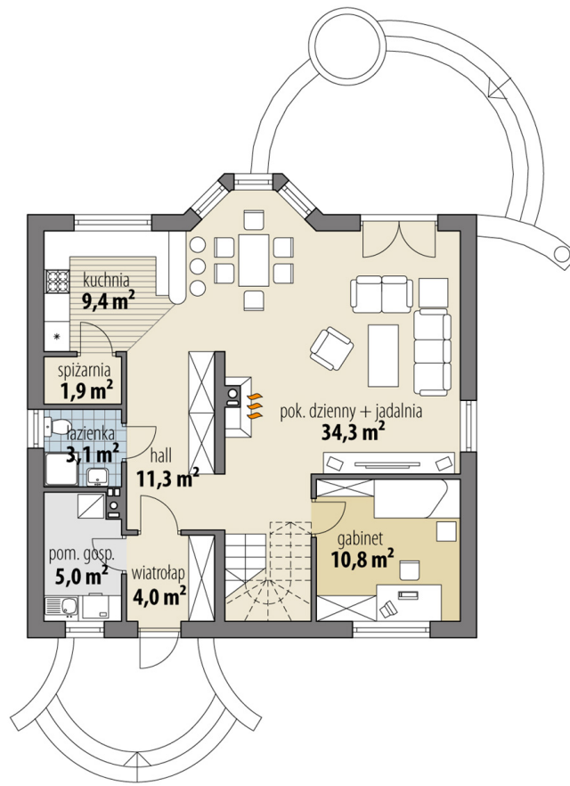
RZUT PARTER
