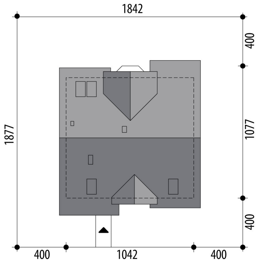
RZUT DZIAŁKI
