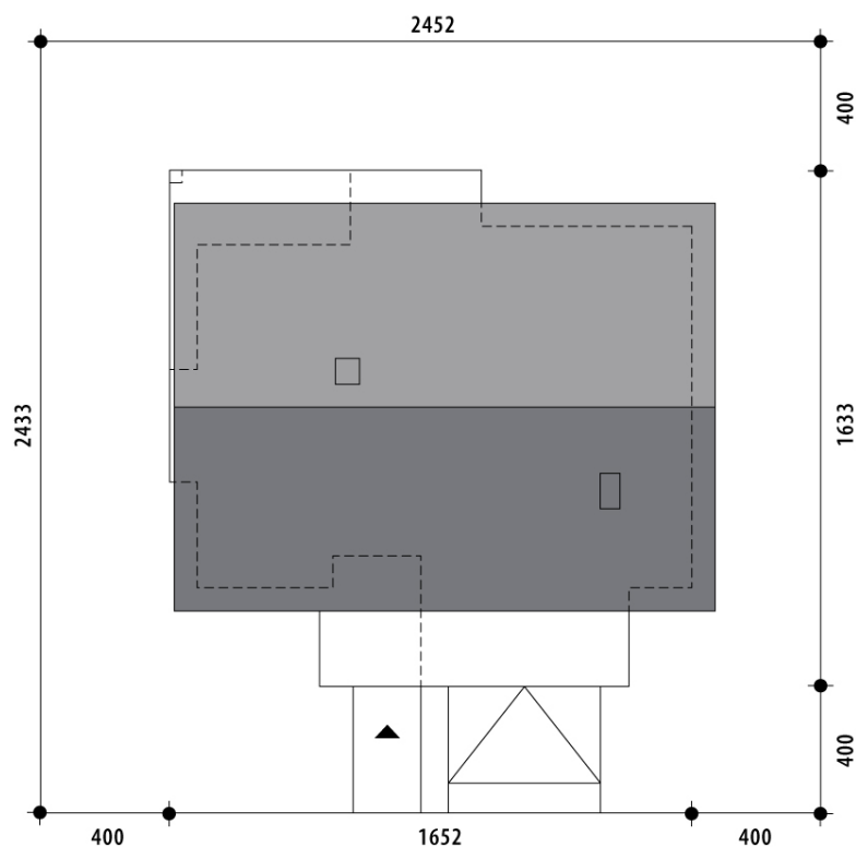
RZUT DZIAŁKI
