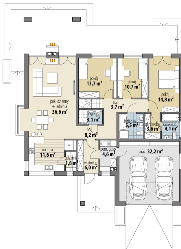
RZUT PARTER
