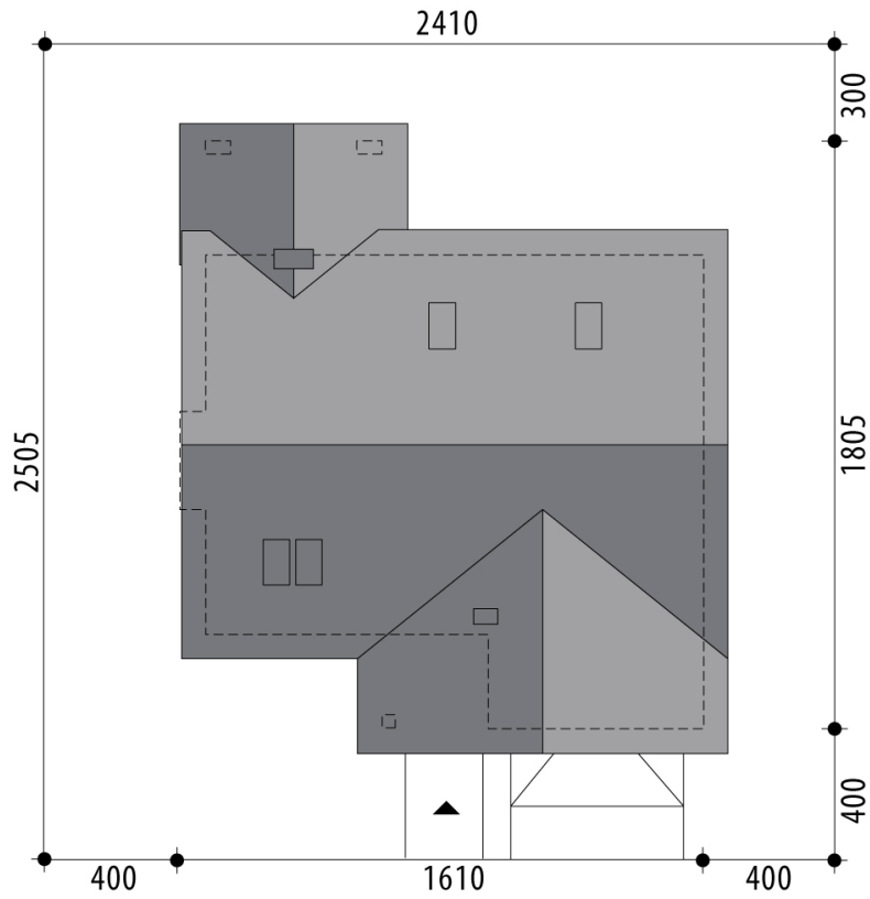
RZUT DZIAŁKI
