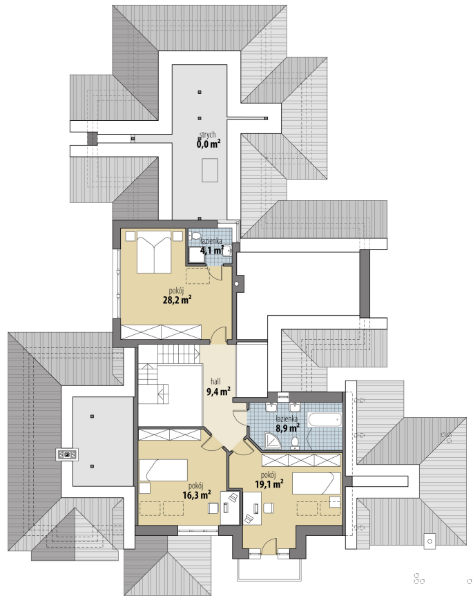
RZUT
