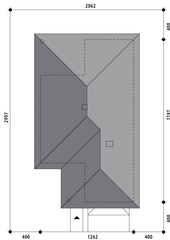
RZUT DZIAŁKI
