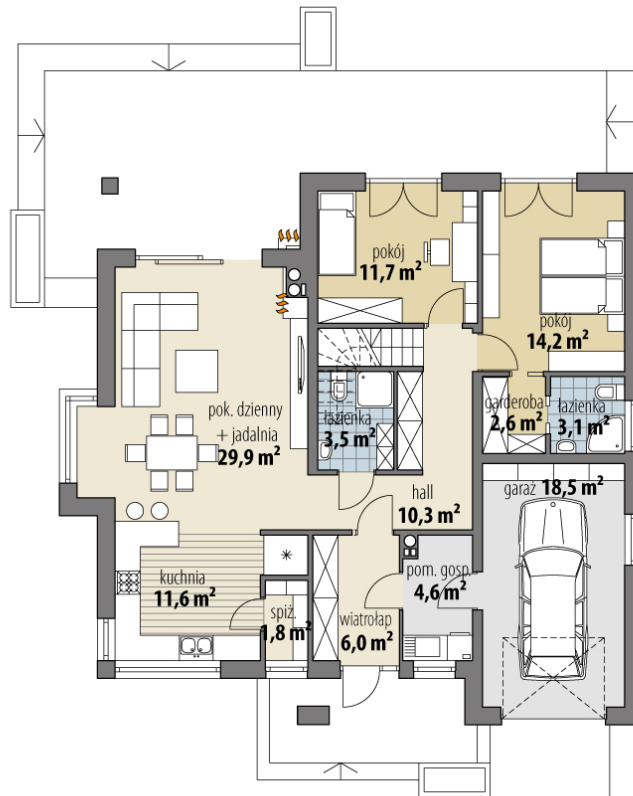
RZUT PARTER
