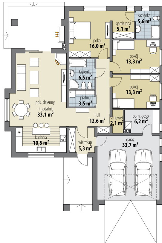
RZUT PARTER
