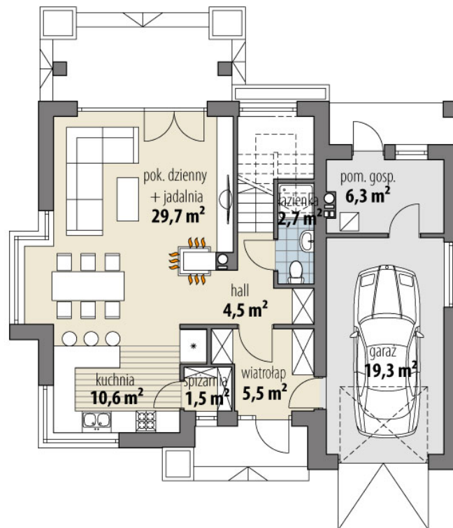
RZUT PARTER
