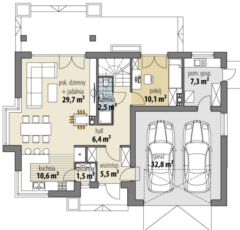
RZUT PARTER
