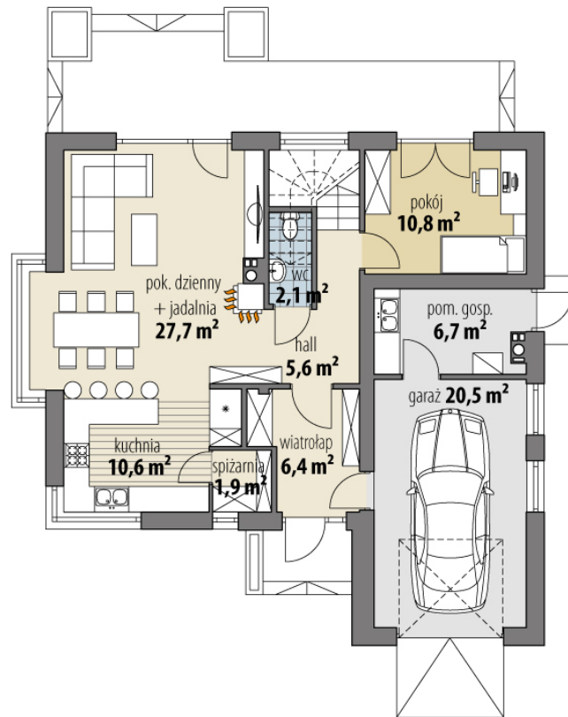
RZUT PARTER
