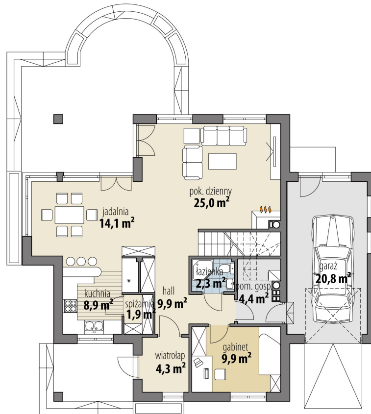
RZUT PARTER
