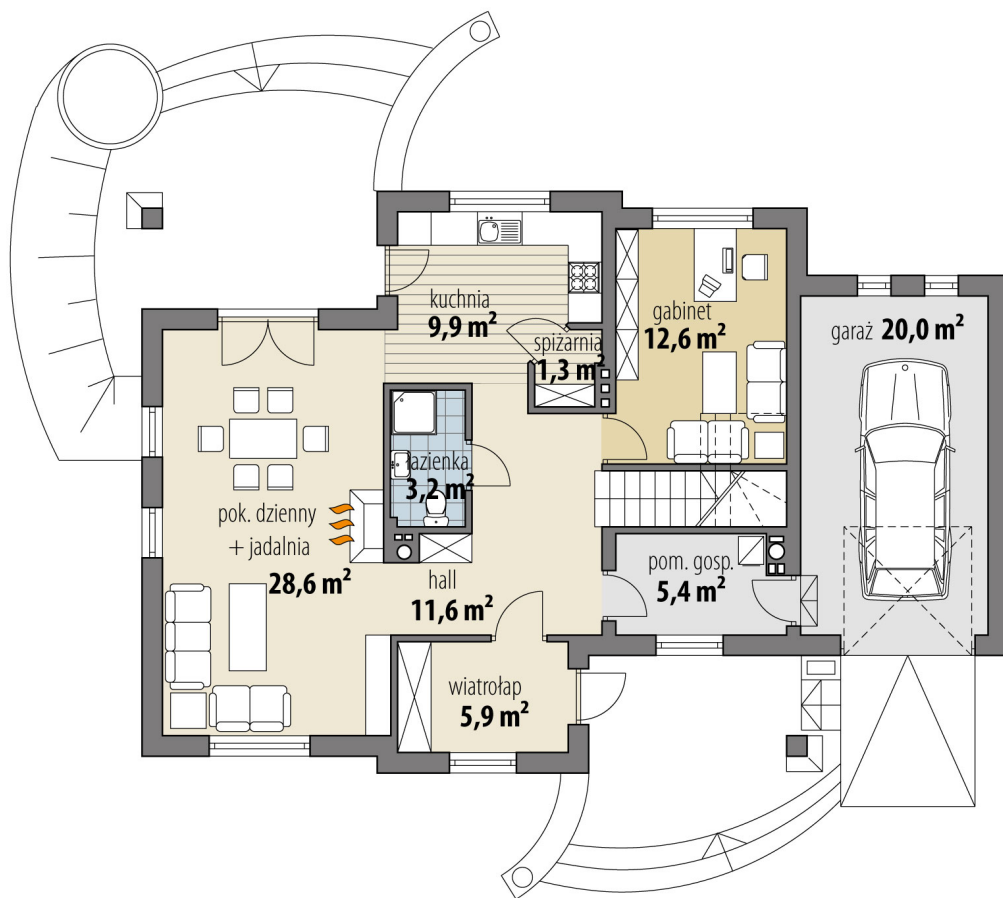
RZUT PARTER
