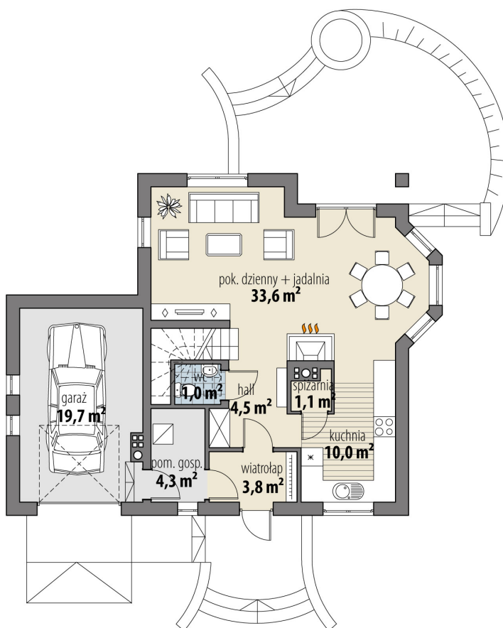
RZUT PARTER
