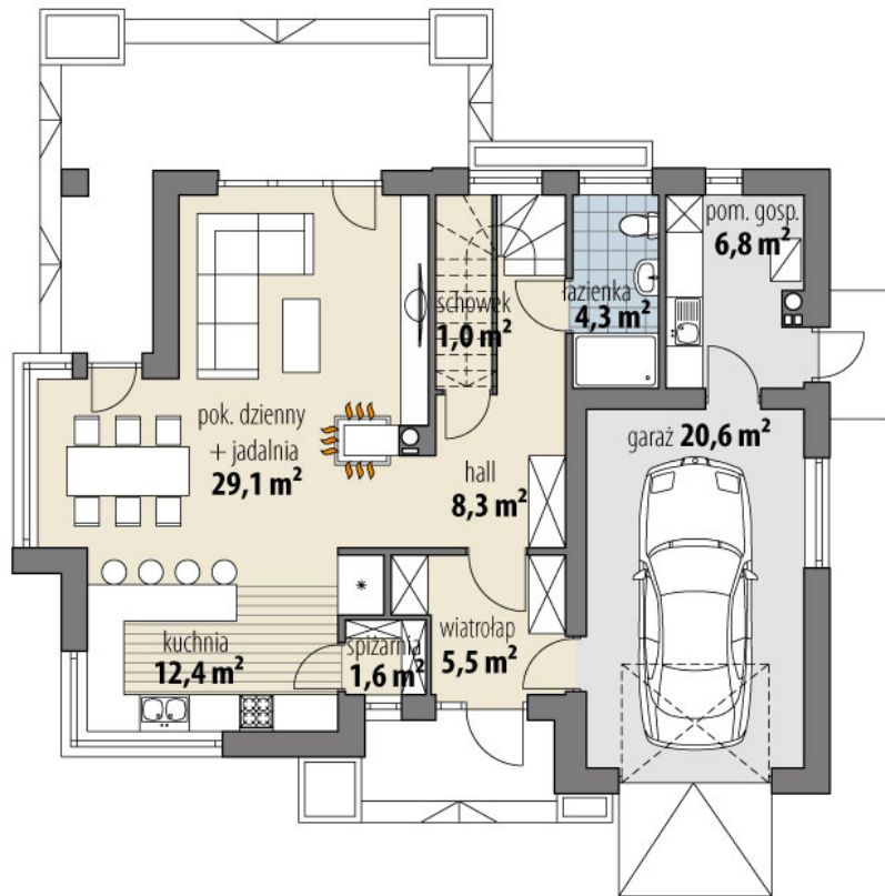
RZUT PARTER
