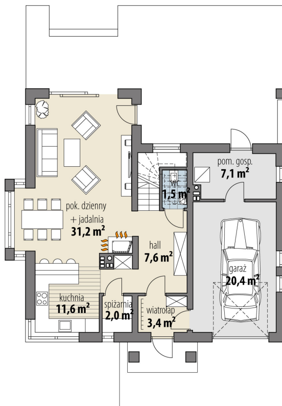
RZUT PARTER
