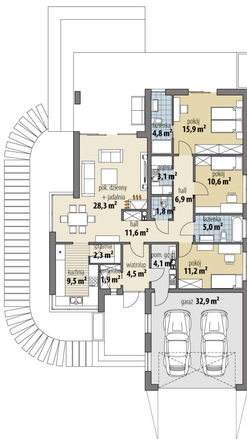
RZUT PARTER
