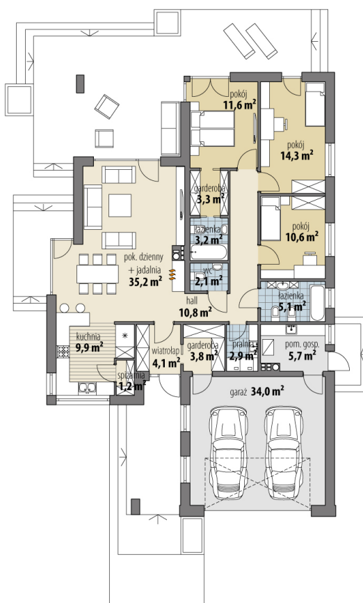
RZUT PARTER
