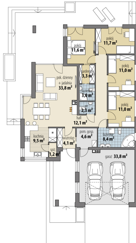
RZUT PARTER
