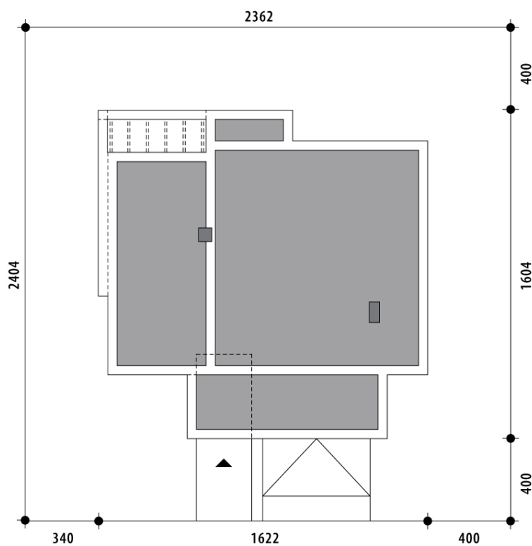
RZUT DZIAŁKI
