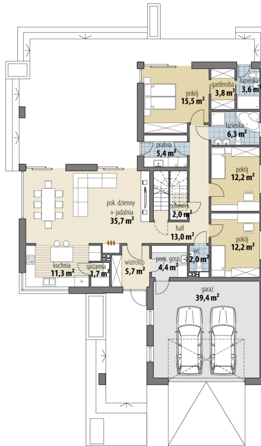
RZUT PARTER
