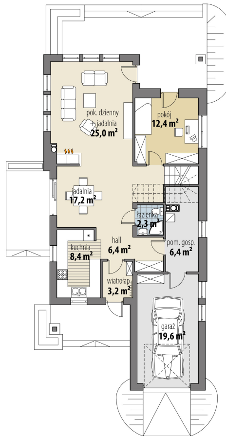
RZUT PARTER
