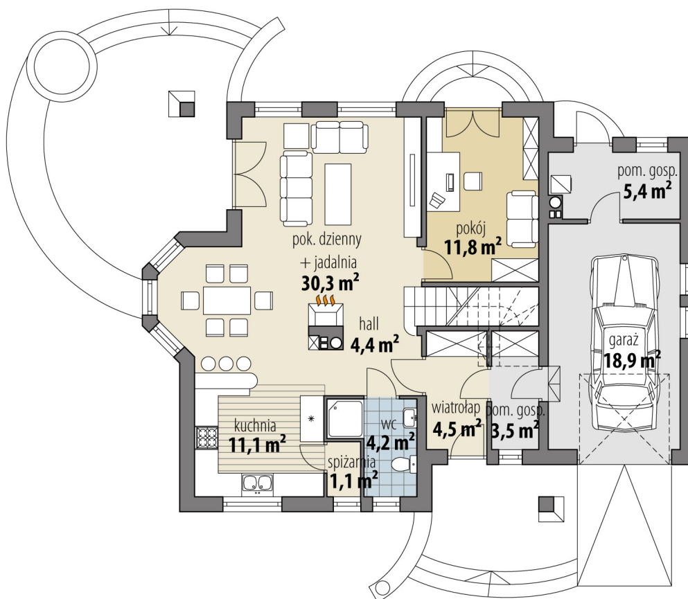
RZUT PARTER
