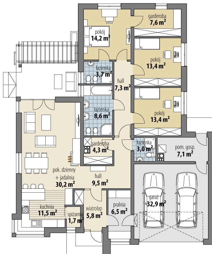
RZUT PARTER
