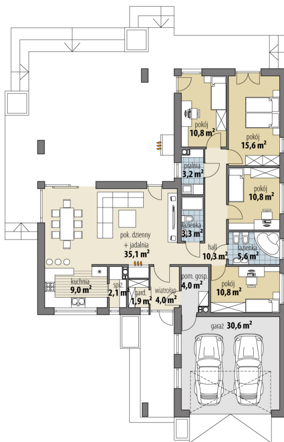
RZUT PARTER
