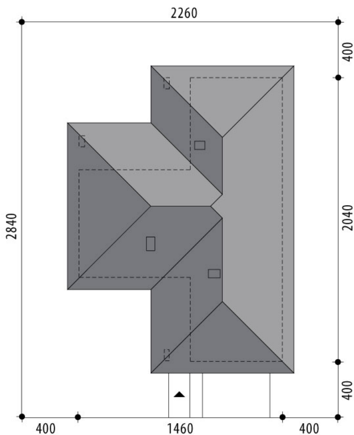
RZUT DZIAŁKI
