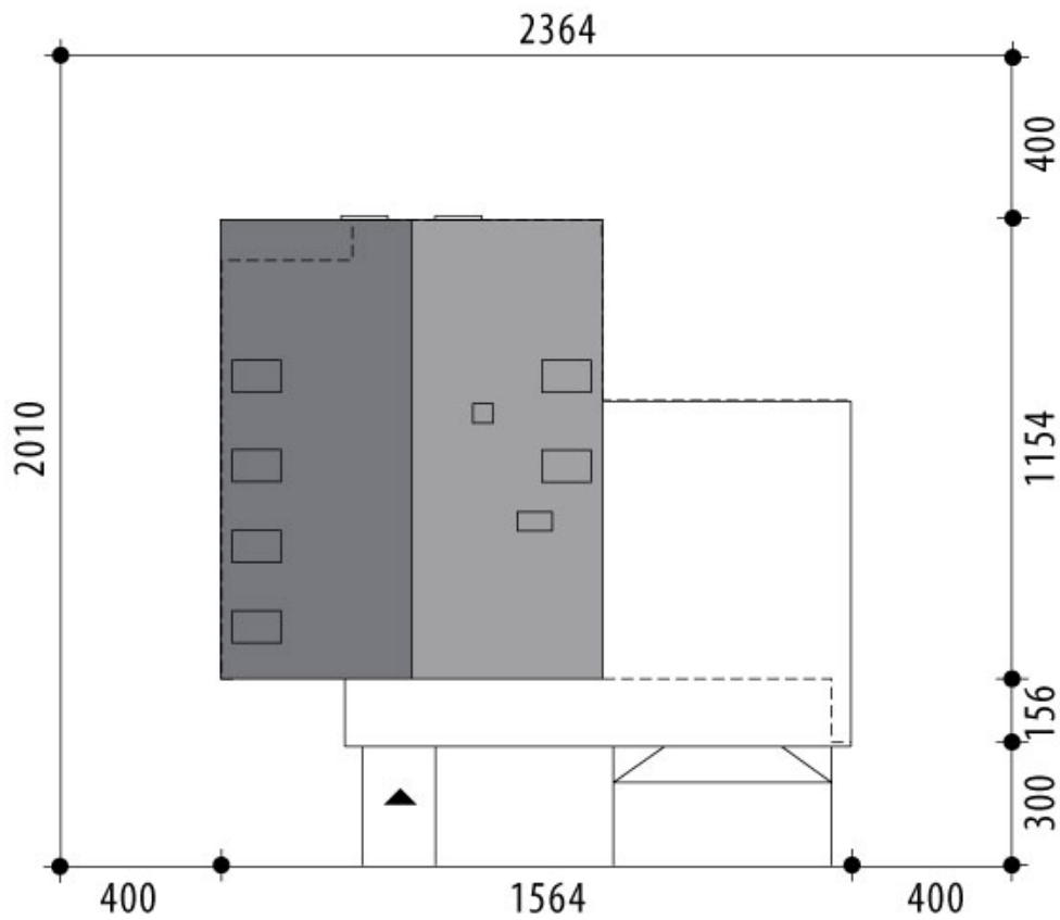
RZUT DZIAŁKI
