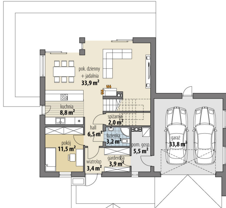
RZUT PARTER
