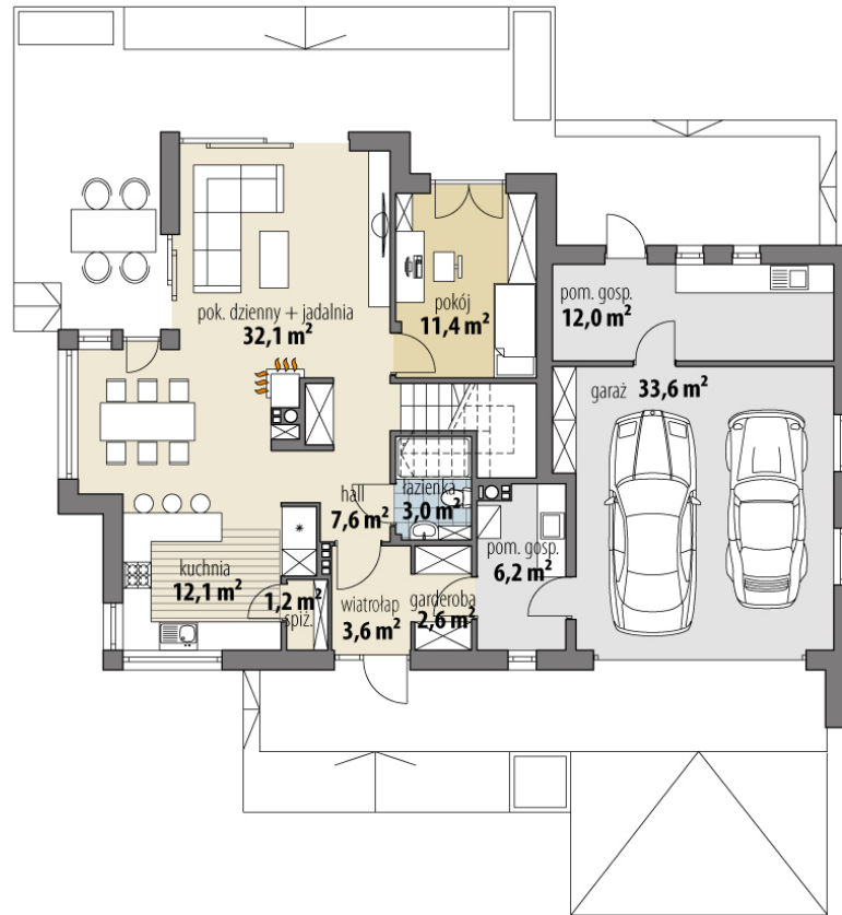
RZUT PARTER
