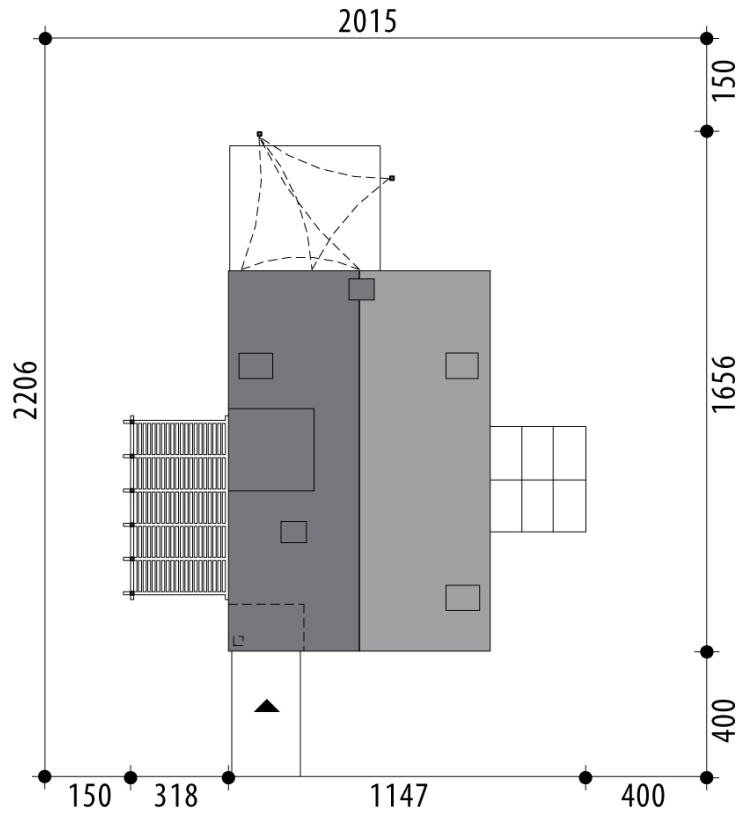
RZUT DZIAŁKI
