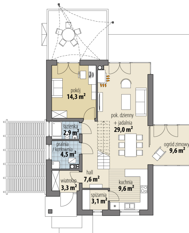
RZUT PARTER
