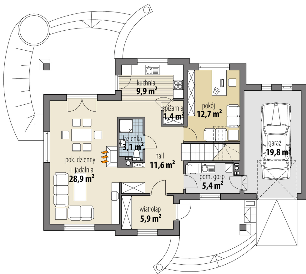
RZUT PARTER
